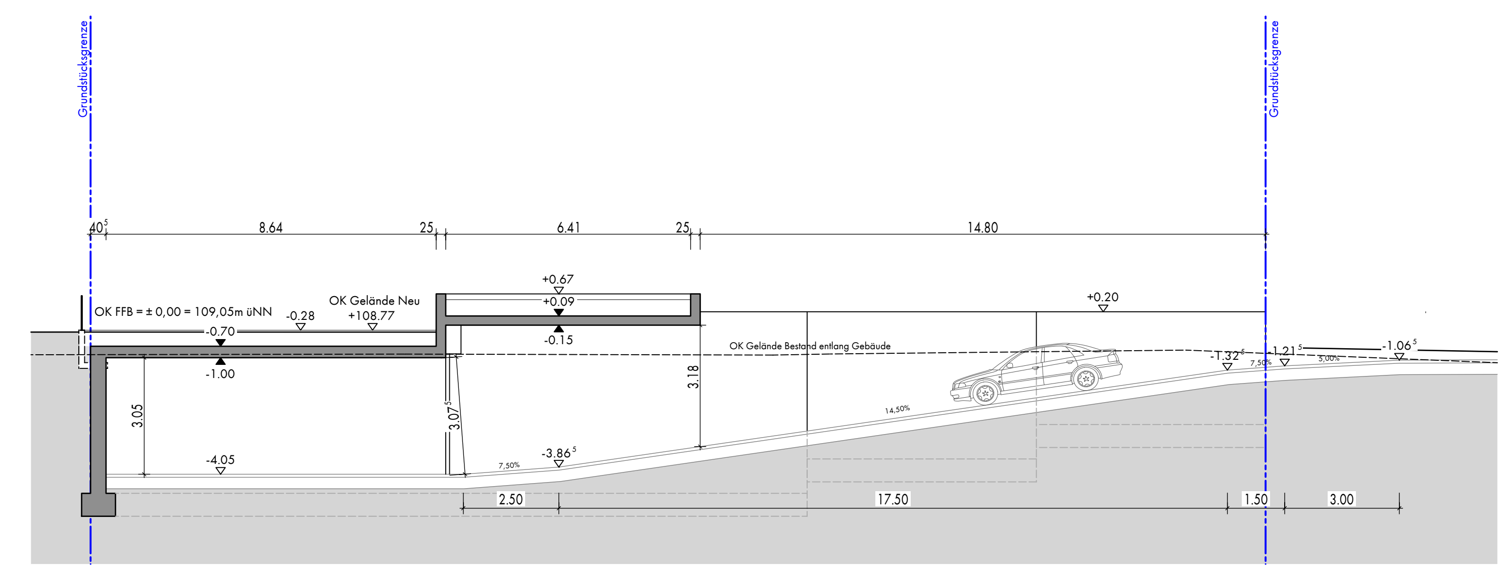
Schnitt A-A
